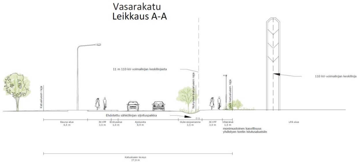
Poikkileikkaus katusuunnitelmasta
